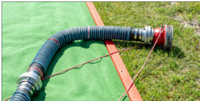
Abb. 37: Richtiges Ablegen des Saugkorbes jenseits der Wassermarkierung (LFV Tirol)
