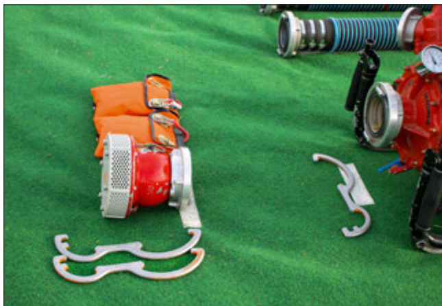
Abb. 7: Auflegen der Bewerbsgeräte Schlüssel, Saugkorb und Leinenbeutel (BFKDO Oberwart)
